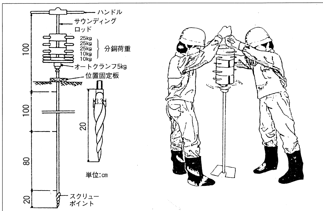
図-2. スウェーデン式サウンディング試験
