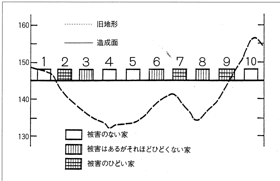
図-1. 造成地盤の不等沈下と旧地形の相関性
